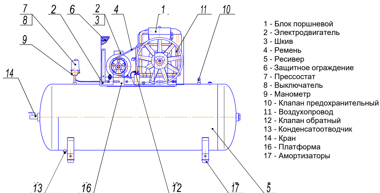
Рисунок 10 - Общий вид компрессора СБ4/Ф-500.AB858/16
