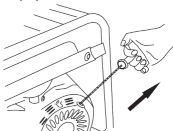
Ручка стартера
