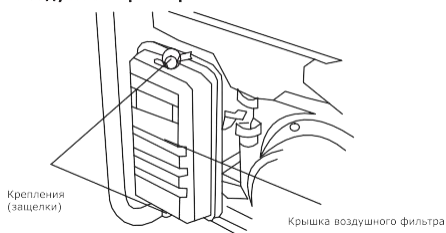
Воздушный фильтр
