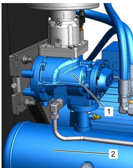
Рис. 11: Ступень компрессора
