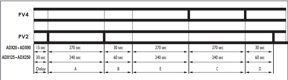
Рис. 2.3.2 Циклограмма открытия и закрытия электромагнитных пневматических клапанов (PV)
