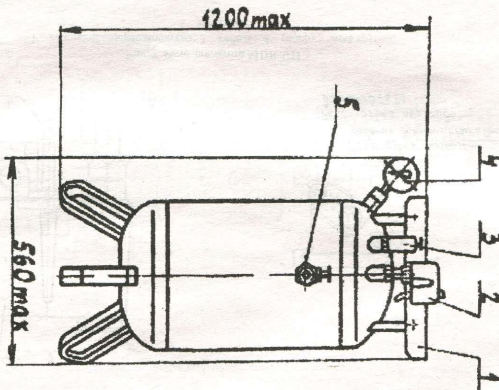
Рис. 6. Ресивер установки компрессорной, модель КВ-7 1 – плита; 2 – реле давления; 3 – клапан предохранительный; 4 – манометр контроля воздуха; 5 – вентиль раздаточный.
