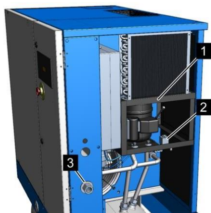
Рис. 23: Рефрижераторный осушитель
